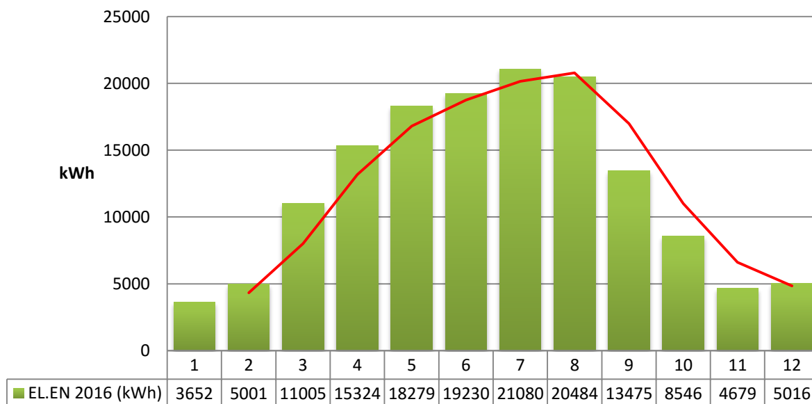
SLIKA: PROIZVEDENA EL.ENERGIJA ( 145.771,00 kWh) u 2016 godini
