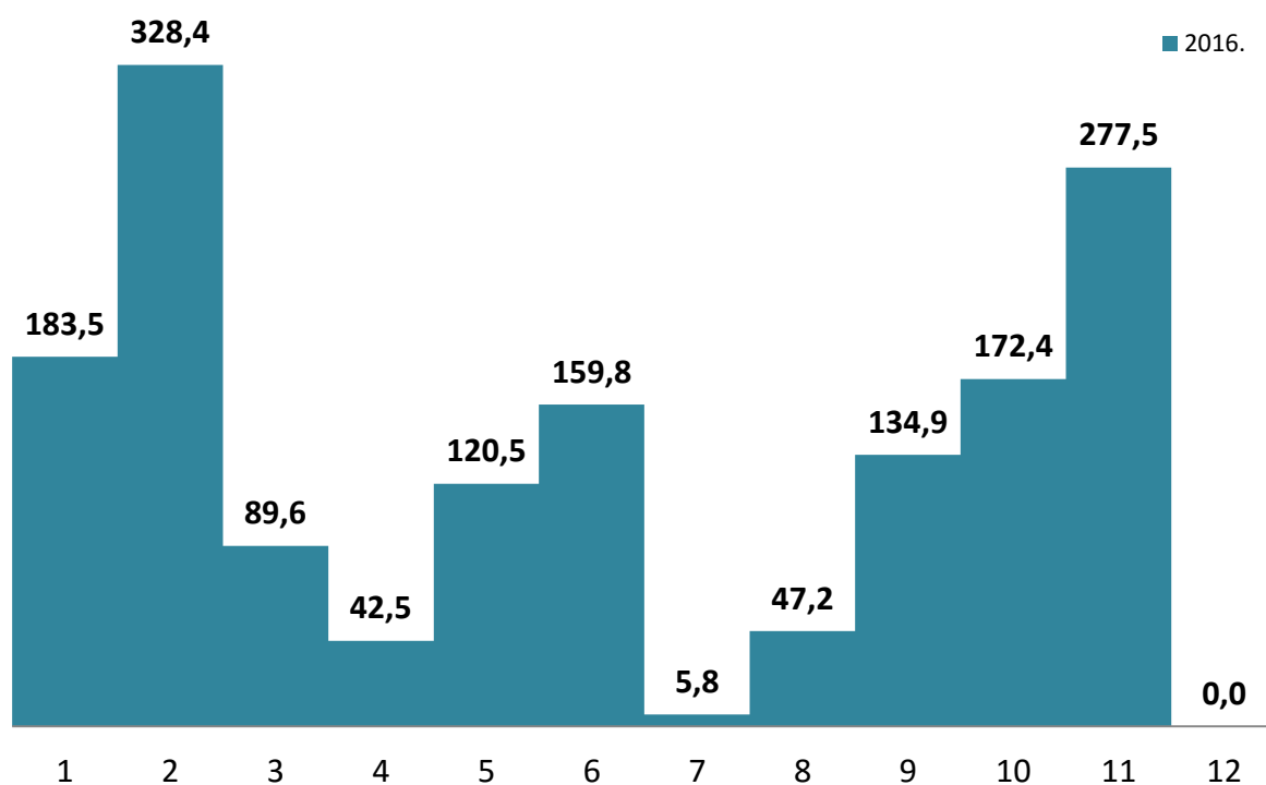
SLIKA: KOLIČINA OBORINA MJERENO NA IZVORIŠTU PONIKVE 2016.G. (l/m 2 )
