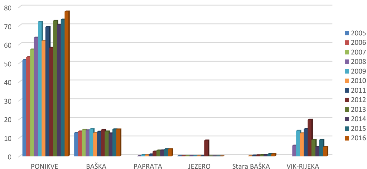
SLIKA: ZAHVAĆENE I PREUZETE KOLIČINE VODE – PROSJEČNO l/s/dan
